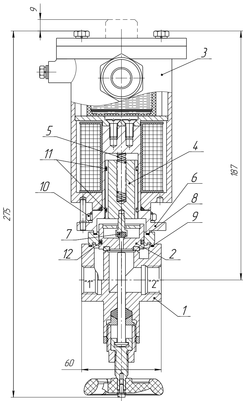
Рис. 2. Клапан муфтовый. Общий вид
